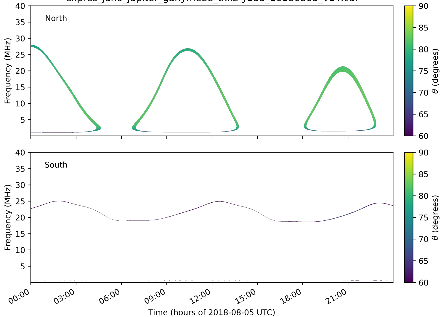
expres_juno_jupiter_ganymede_txka-y235_20180805_v14.cdf
