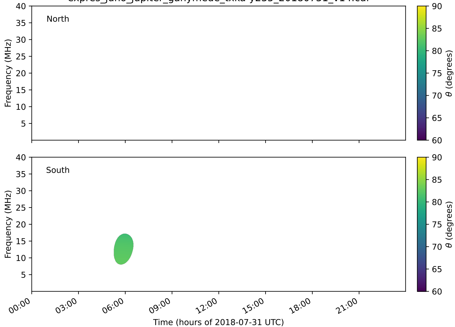
expres_juno_jupiter_ganymede_txka-y235_20180731_v14.cdf
