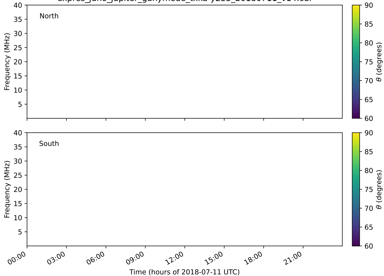
expres_juno_jupiter_ganymede_txka-y235_20180711_v14.cdf
