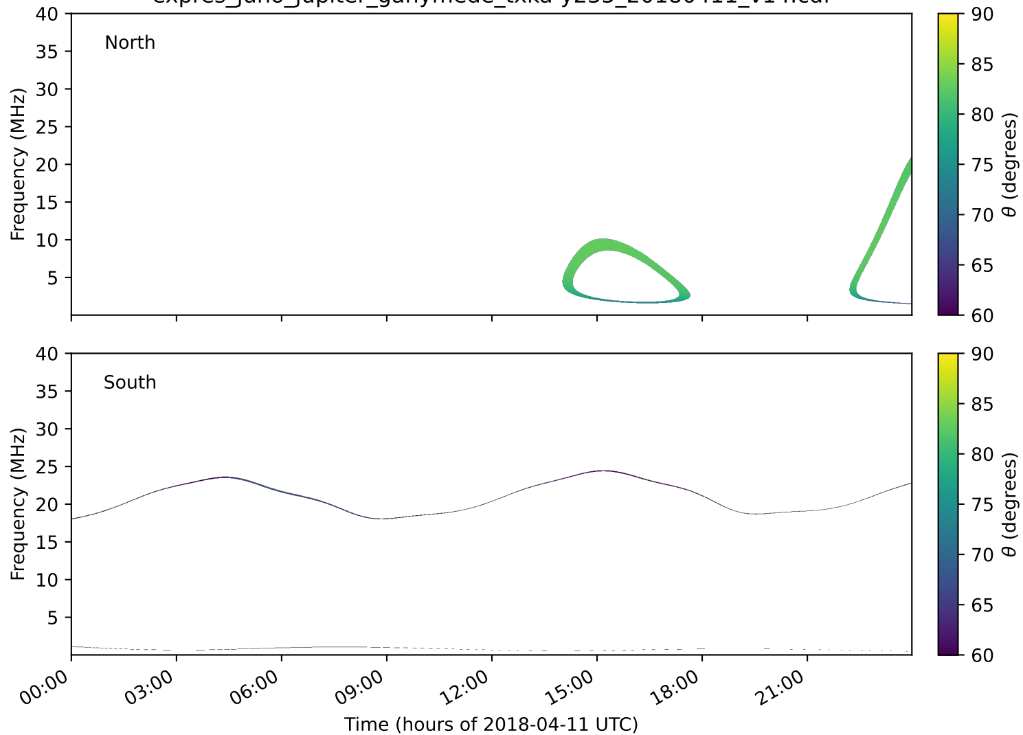
expres_juno_jupiter_ganymede_txka-y235_20180411_v14.cdf
