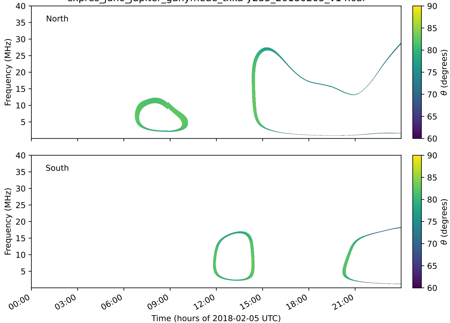
expres_juno_jupiter_ganymede_txka-y235_20180205_v14.cdf
