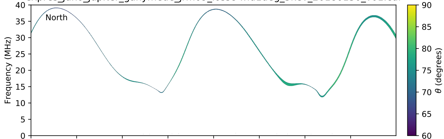
expres_juno_jupiter_ganymede_jrm09_lossc-wid1deg_3kev_20180130_v01.cdf
