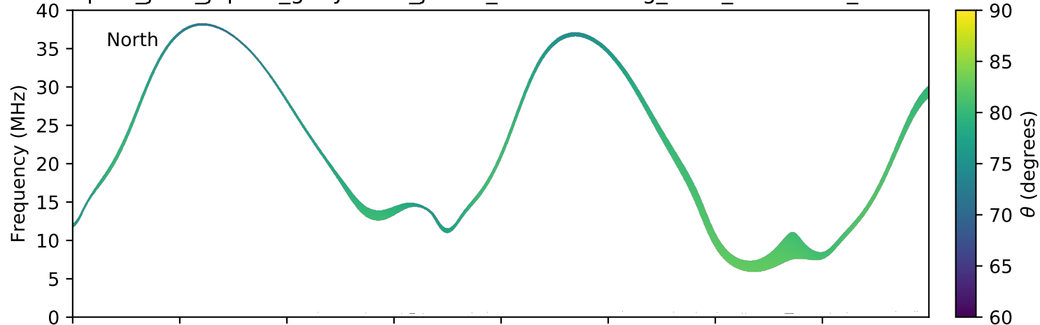
expres_juno_jupiter_ganymede_jrm09_lossc-wid1deg_3kev_20180120_v01.cdf
