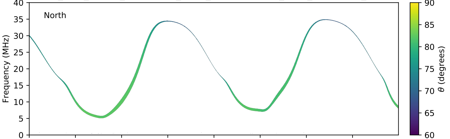
expres_juno_jupiter_ganymede_isaac_lossc-wid1deg_3kev_20180109_v01.cdf
