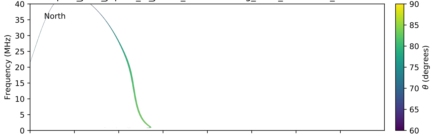
expres_juno_jupiter_io_jrm09_lossc-wid1deg_3kev_20171201_v01.cdf
