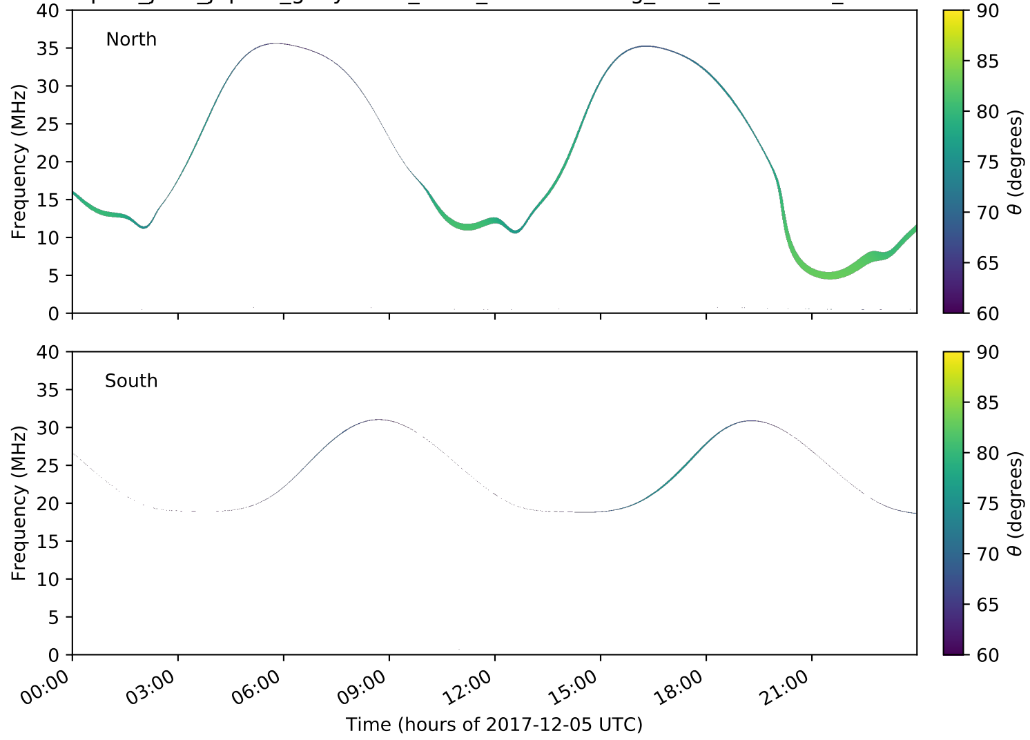
expres_juno_jupiter_ganymede_isaac_lossc-wid1deg_3kev_20171205_v01.cdf
