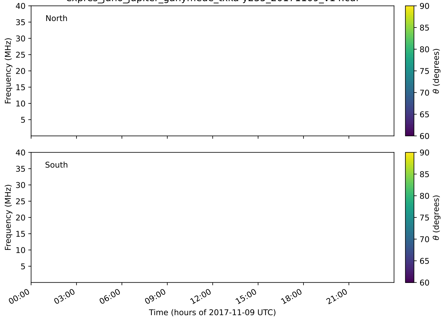
expres_juno_jupiter_ganymede_txka-y235_20171109_v14.cdf
