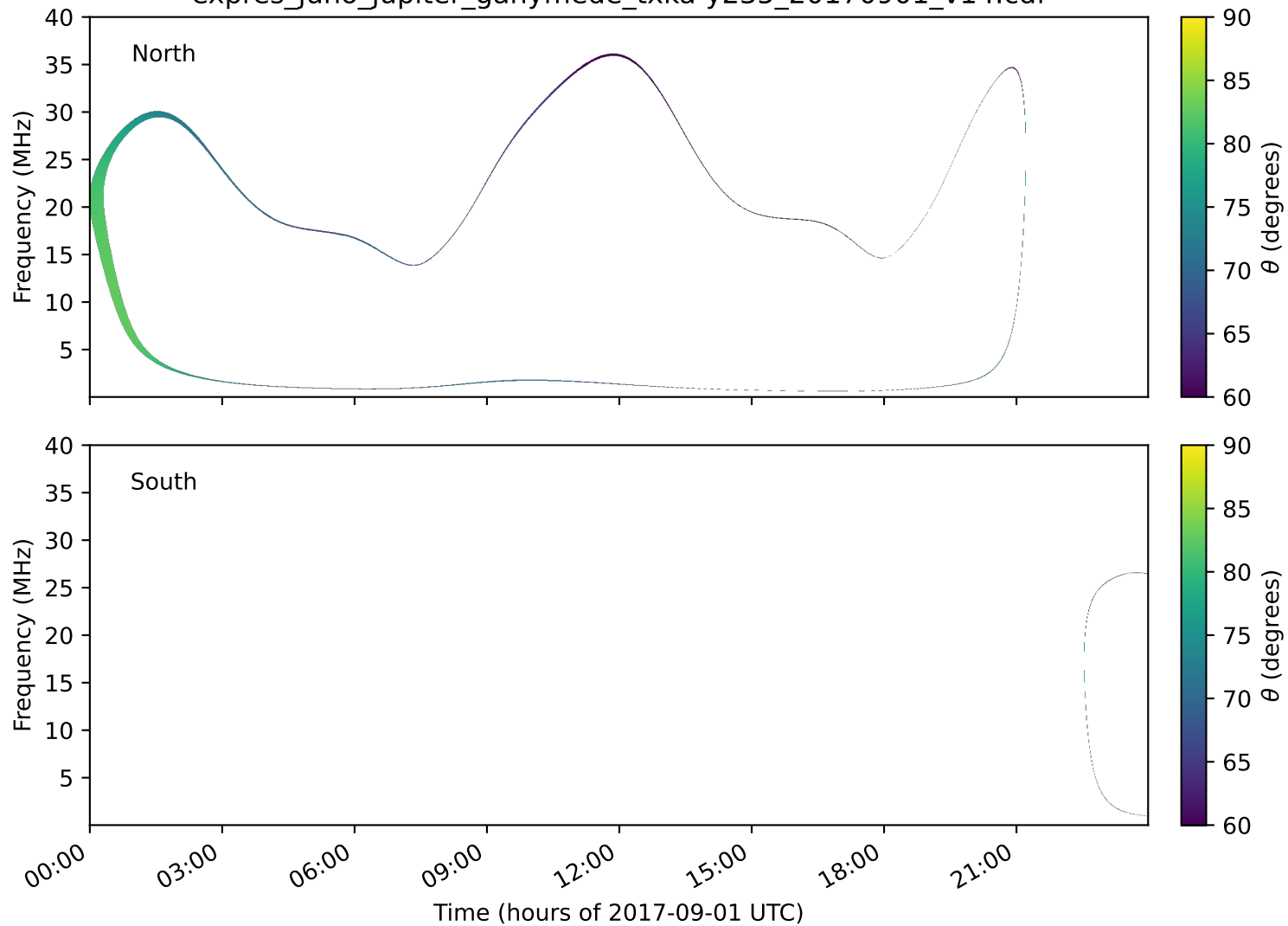
expres_juno_jupiter_ganymede_txka-y235_20170901_v14.cdf
