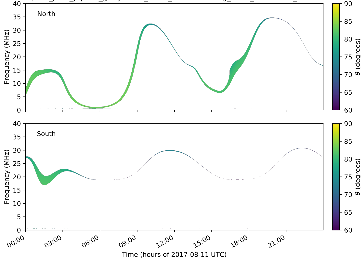
expres_juno_jupiter_ganymede_isaac_lossc-wid1deg_3kev_20170811_v01.cdf
