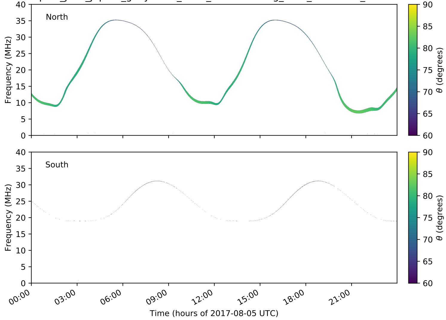
expres_juno_jupiter_ganymede_isaac_lossc-wid1deg_3kev_20170805_v01.cdf
