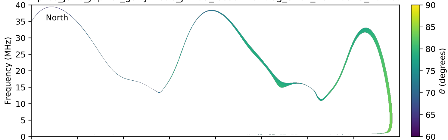
expres_juno_jupiter_ganymede_jrm09_lossc-wid1deg_3kev_20170323_v01.cdf
