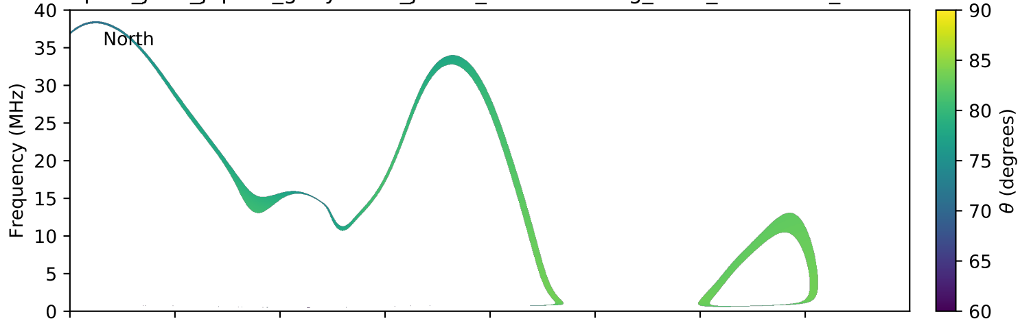
expres_juno_jupiter_ganymede_jrm09_lossc-wid1deg_3kev_20170316_v01.cdf
