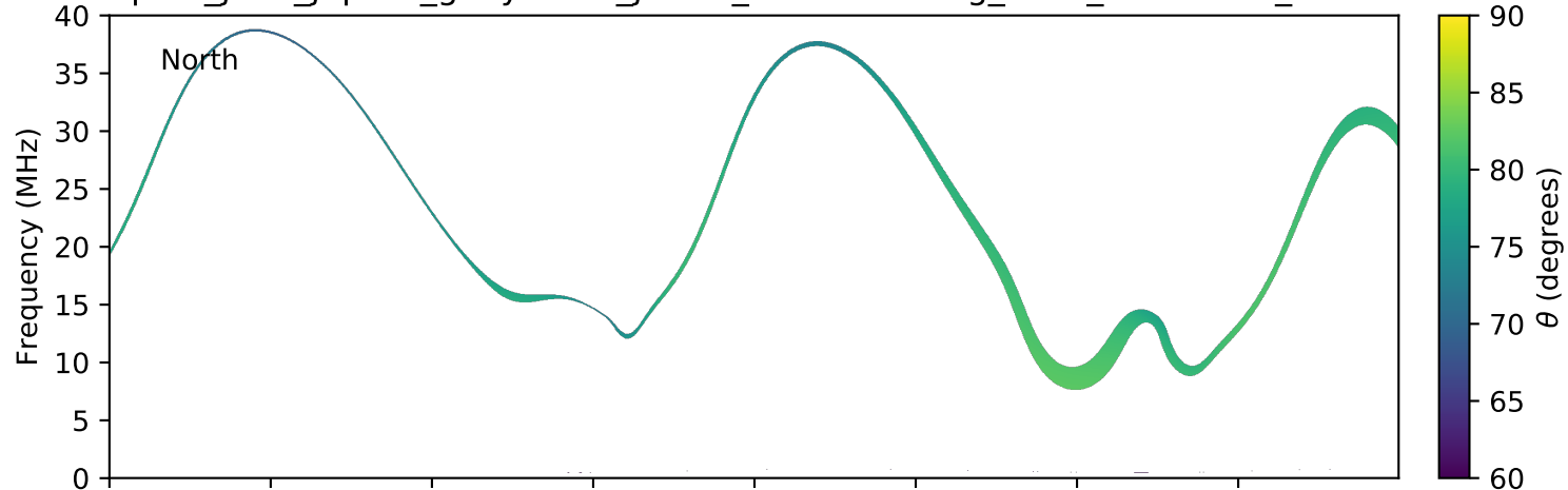
expres_juno_jupiter_ganymede_jrm09_lossc-wid1deg_3kev_20170301_v01.cdf
