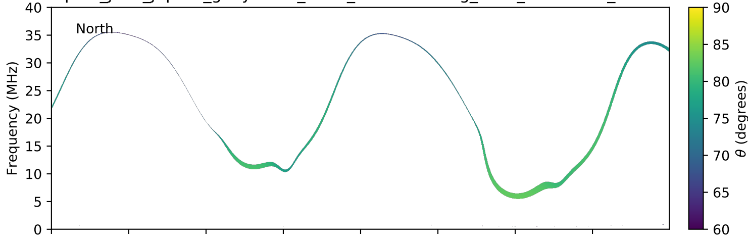
expres_juno_jupiter_ganymede_isaac_lossc-wid1deg_3kev_20170301_v01.cdf
