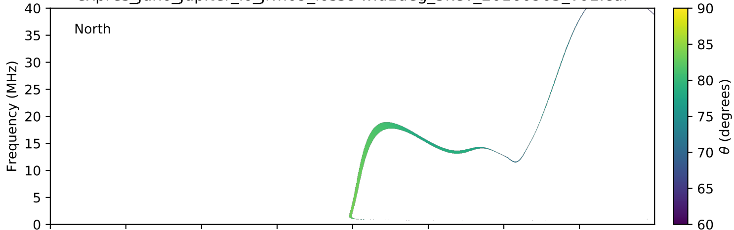
expres_juno_jupiter_io_jrm09_lossc-wid1deg_3kev_20160905_v01.cdf
