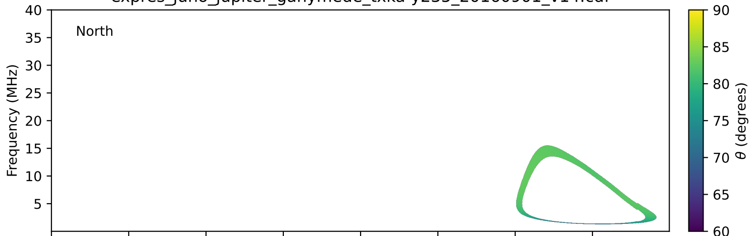
expres_juno_jupiter_ganymede_txka-y235_20160901_v14.cdf
