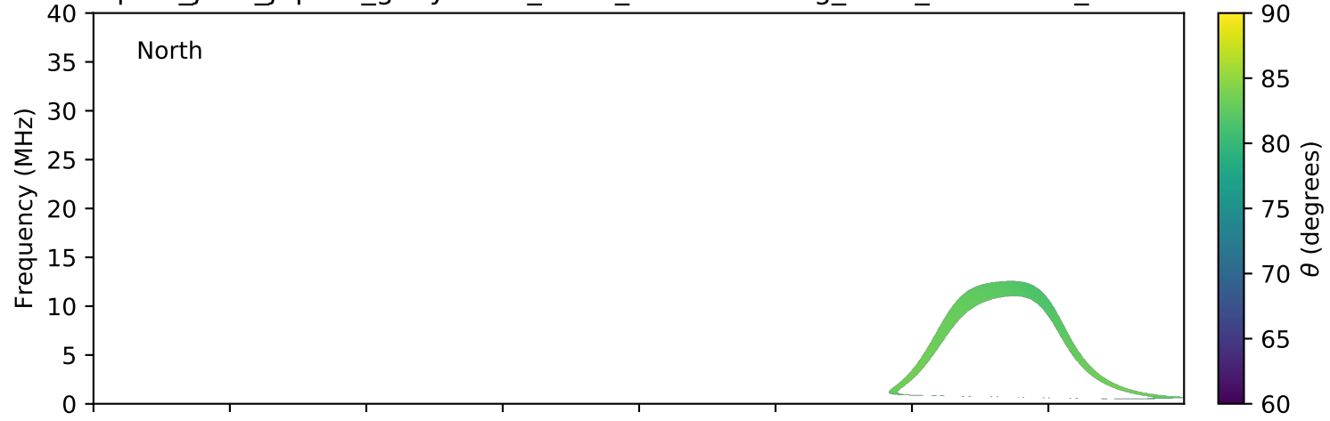
expres_juno_jupiter_ganymede_isaac_lossc-wid1deg_3kev_20160901_v01.cdf
