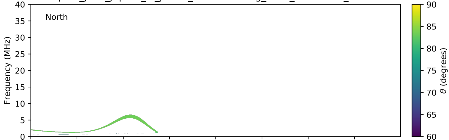
expres_juno_jupiter_io_jrm09_lossc-wid1deg_3kev_20160828_v01.cdf
