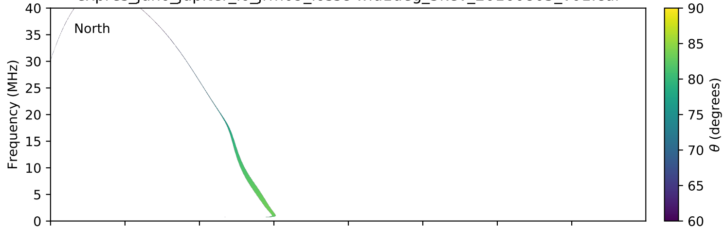
expres_juno_jupiter_io_jrm09_lossc-wid1deg_3kev_20160805_v01.cdf
