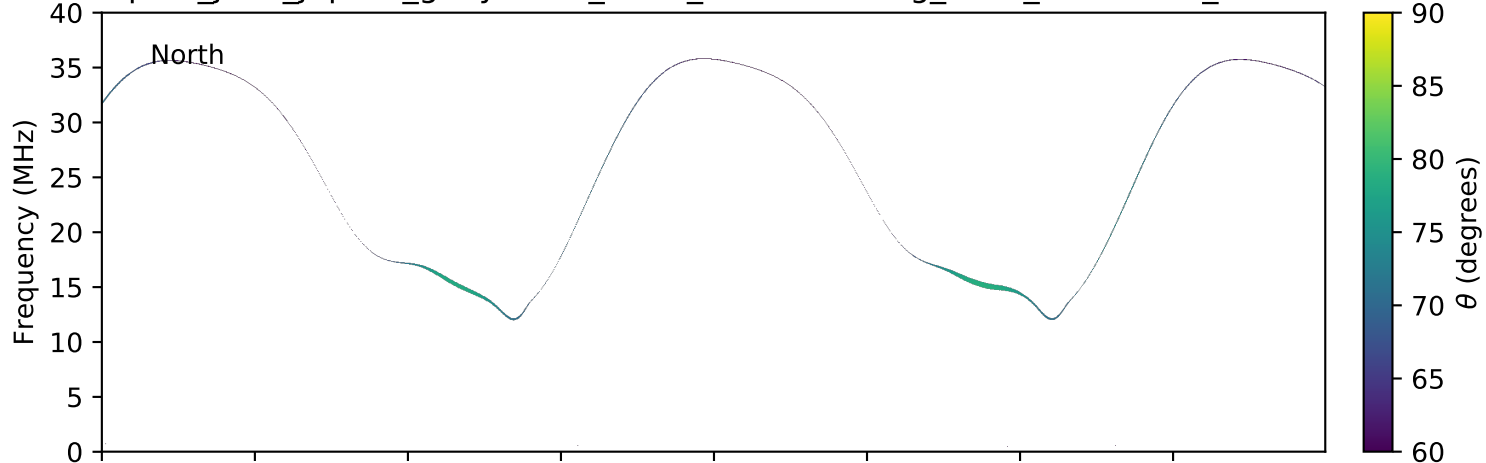
expres_juno_jupiter_ganymede_isaac_lossc-wid1deg_3kev_20160805_v01.cdf
