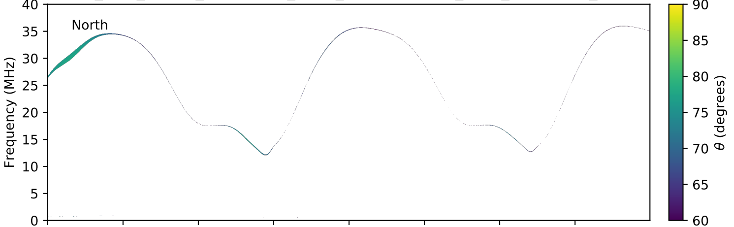
expres_juno_jupiter_ganymede_isaac_lossc-wid1deg_3kev_20160131_v01.cdf
