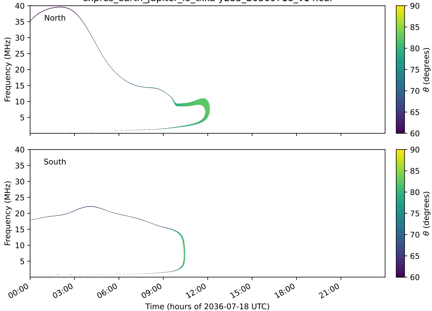
expres_earth_jupiter_io_txka-y235_20360718_v14.cdf
