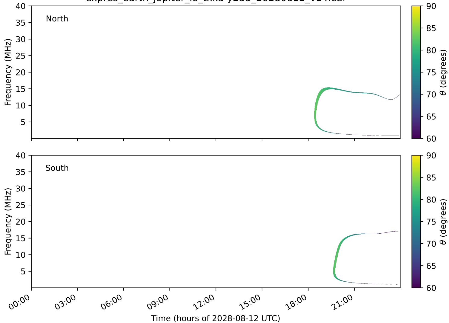
expres_earth_jupiter_io_txka-y235_20280812_v14.cdf
