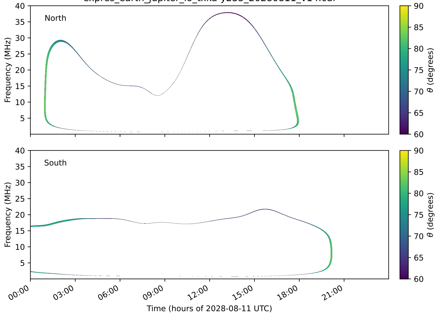
expres_earth_jupiter_io_txka-y235_20280811_v14.cdf
