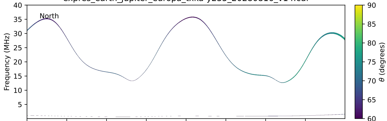
expres_earth_jupiter_europa_txka-y235_20280816_v14.cdf
