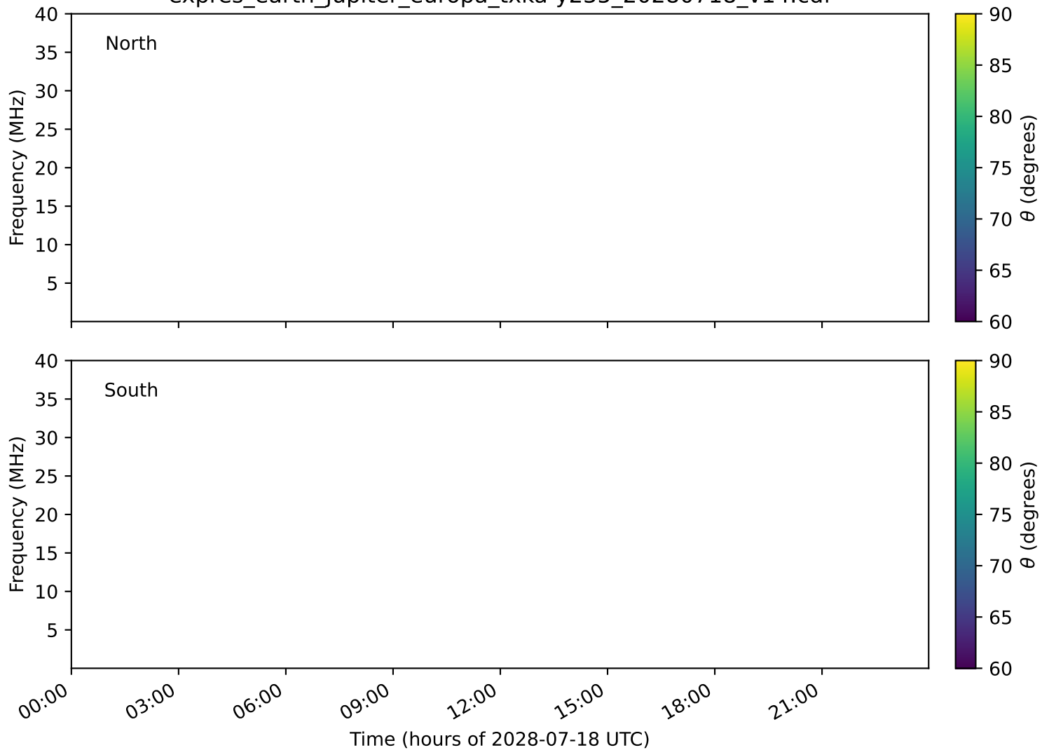
expres_earth_jupiter_europa_txka-y235_20280718_v14.cdf
