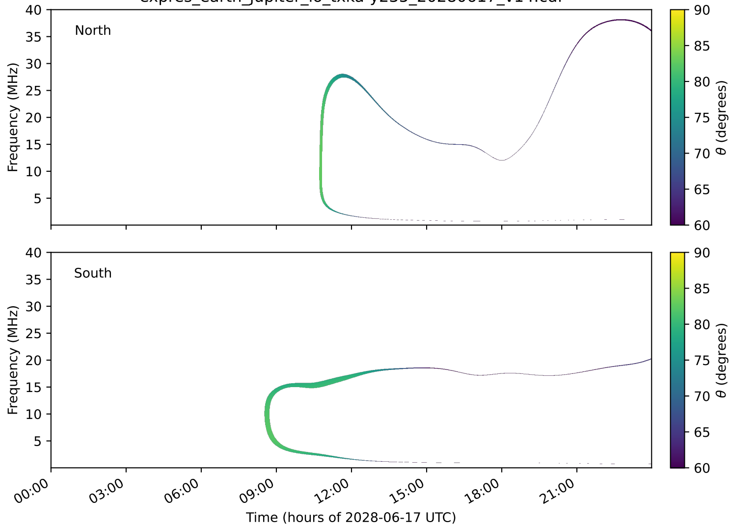
expres_earth_jupiter_io_txka-y235_20280617_v14.cdf
