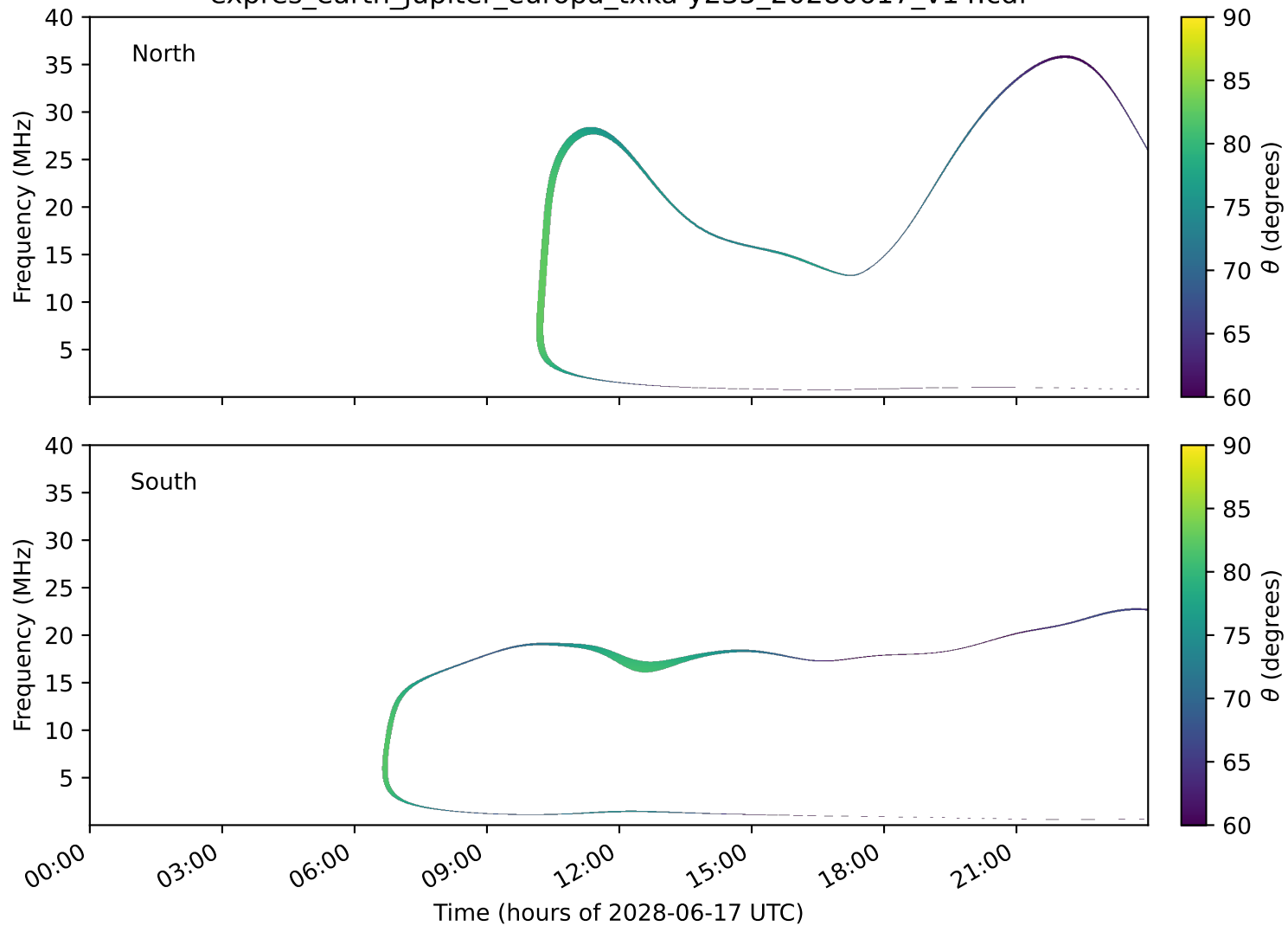
expres_earth_jupiter_europa_txka-y235_20280617_v14.cdf
