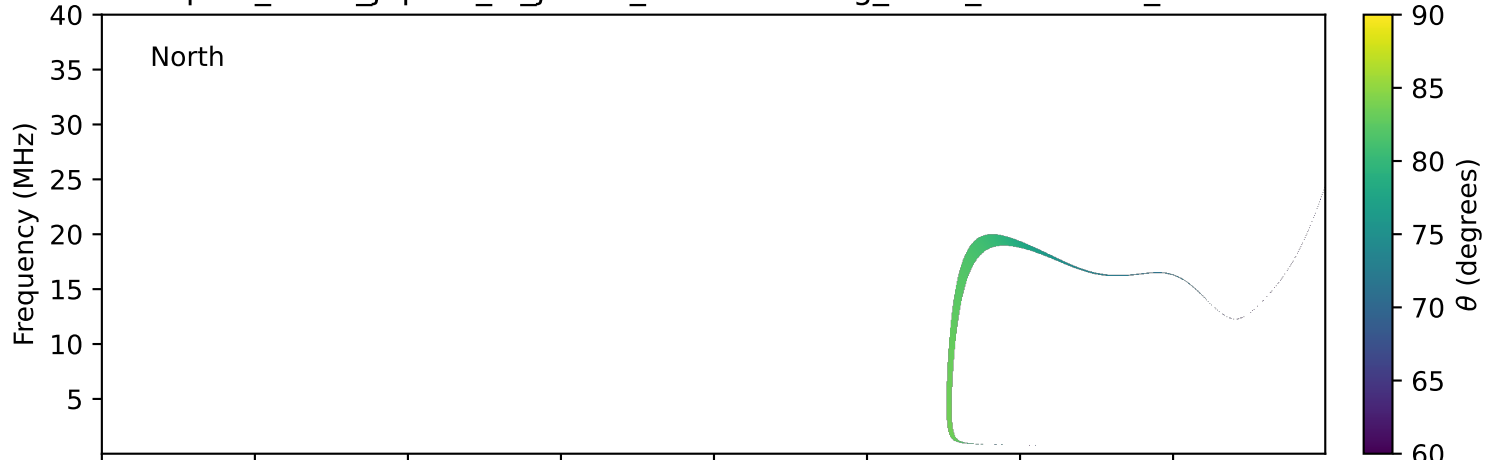
expres_earth_jupiter_io_jrm33_lossc-wid1deg_3kev_20270209_v11.cdf
