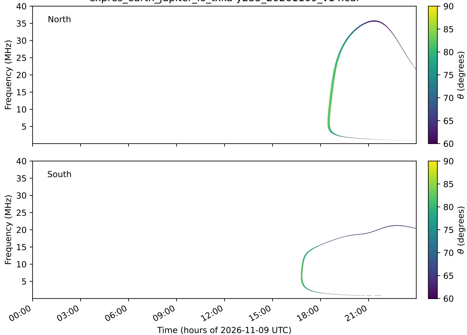
expres_earth_jupiter_io_txka-y235_20261109_v14.cdf
