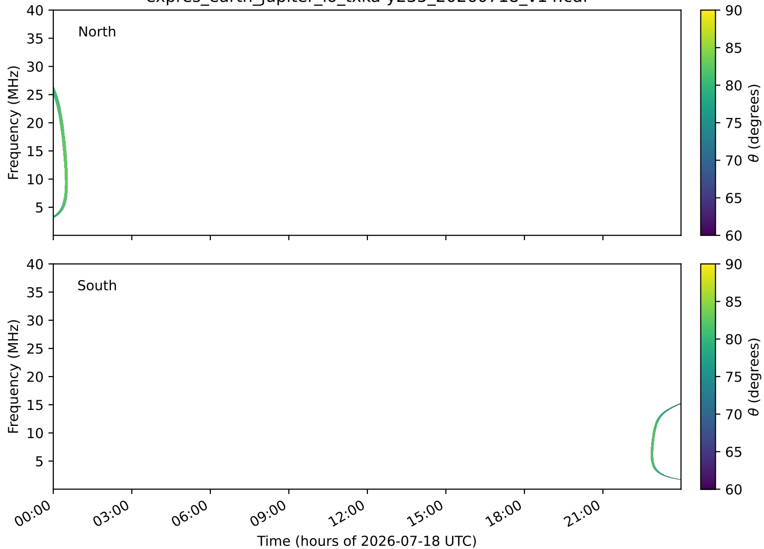
expres_earth_jupiter_io_txka-y235_20260718_v14.cdf
