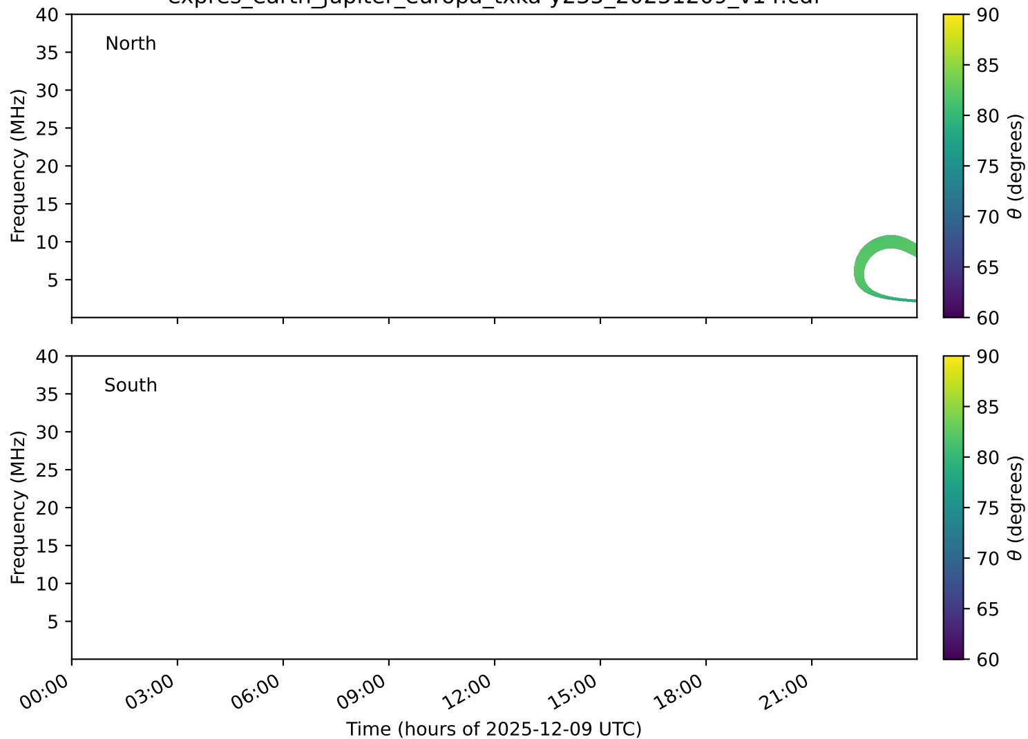
expres_earth_jupiter_europa_txka-y235_20251209_v14.cdf
