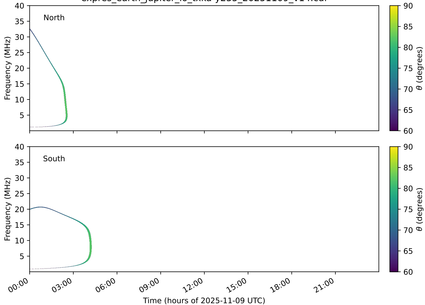
expres_earth_jupiter_io_txka-y235_20251109_v14.cdf
