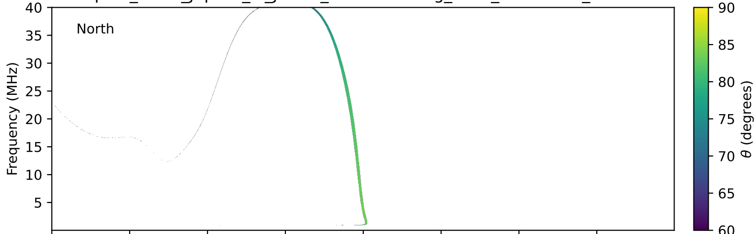
expres_earth_jupiter_io_jrm33_lossc-wid1deg_3kev_20250209_v11.cdf
