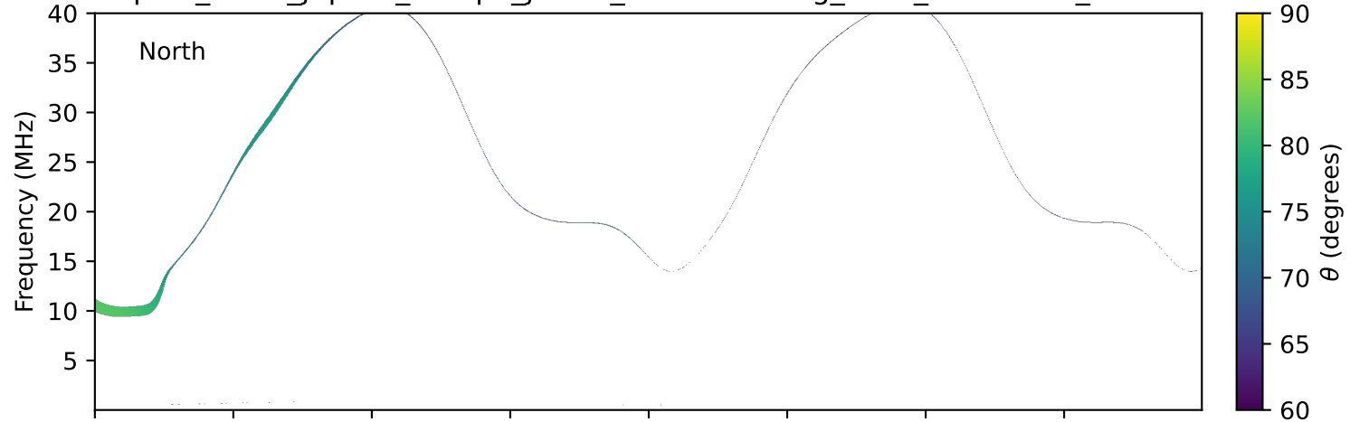
expres_earth_jupiter_europa_jrm33_lossc-wid1deg_3kev_20241209_v11.cdf
