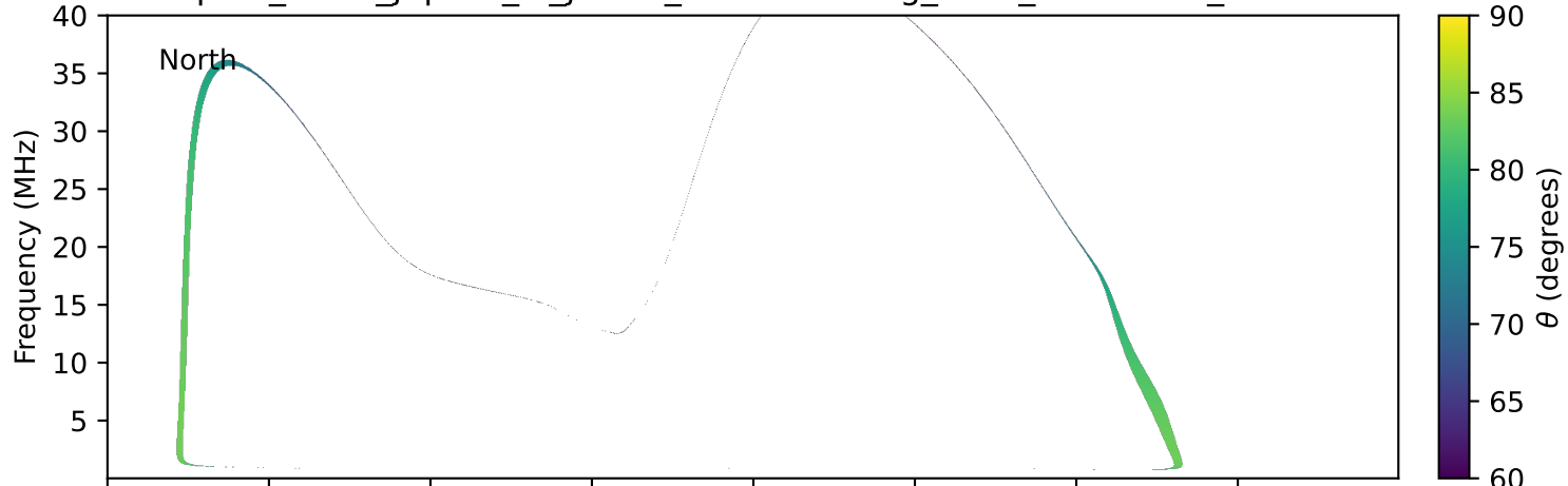
expres_earth_jupiter_io_jrm09_lossc-wid1deg_3kev_20231011_v11.cdf
