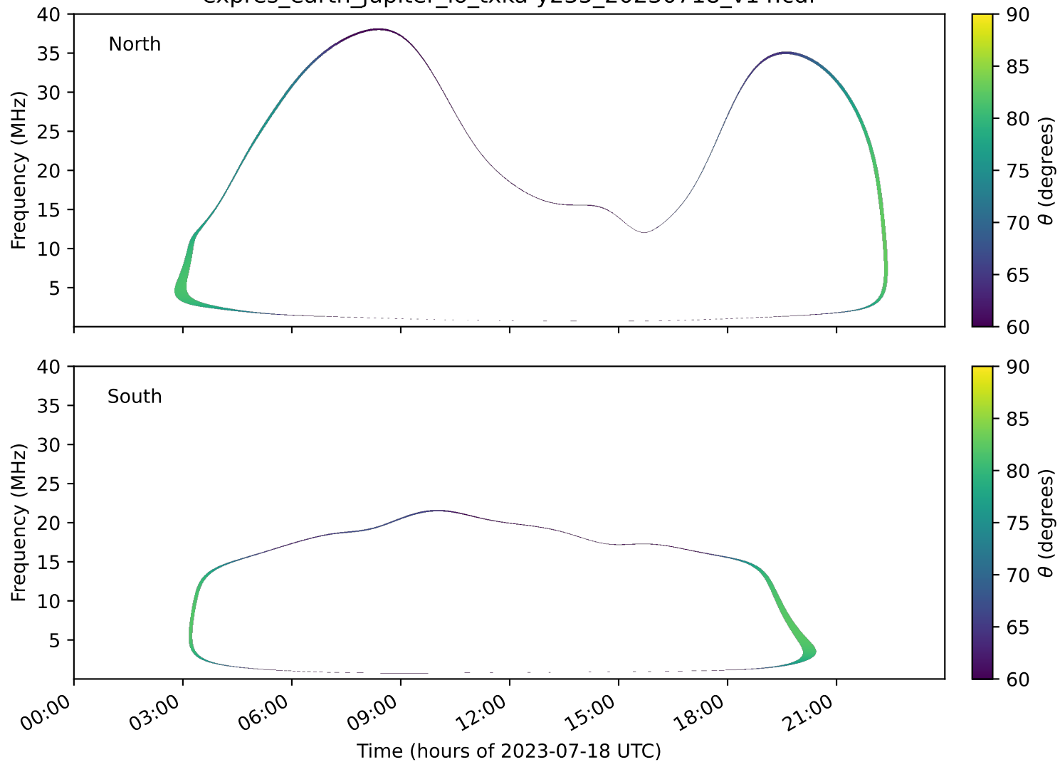
expres_earth_jupiter_io_txka-y235_20230718_v14.cdf
