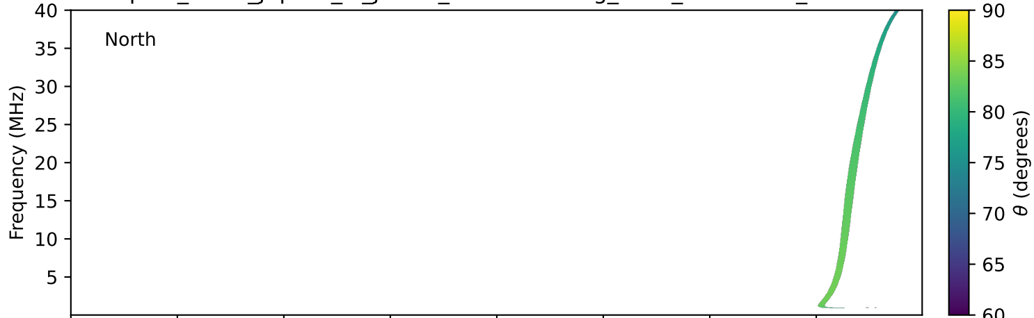
expres_earth_jupiter_io_jrm09_lossc-wid1deg_3kev_20230402_v11.cdf
