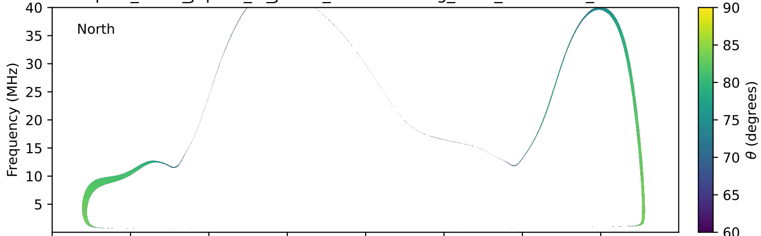
expres_earth_jupiter_io_jrm09_lossc-wid1deg_3kev_20230401_v11.cdf
