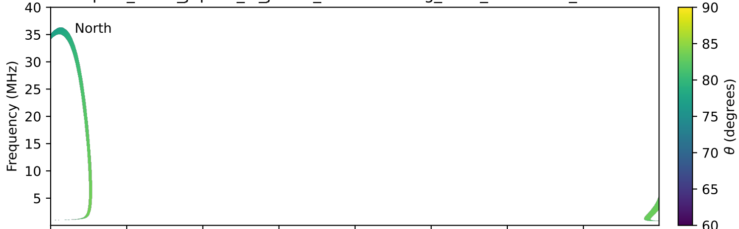
expres_earth_jupiter_io_jrm09_lossc-wid1deg_3kev_20230301_v11.cdf
