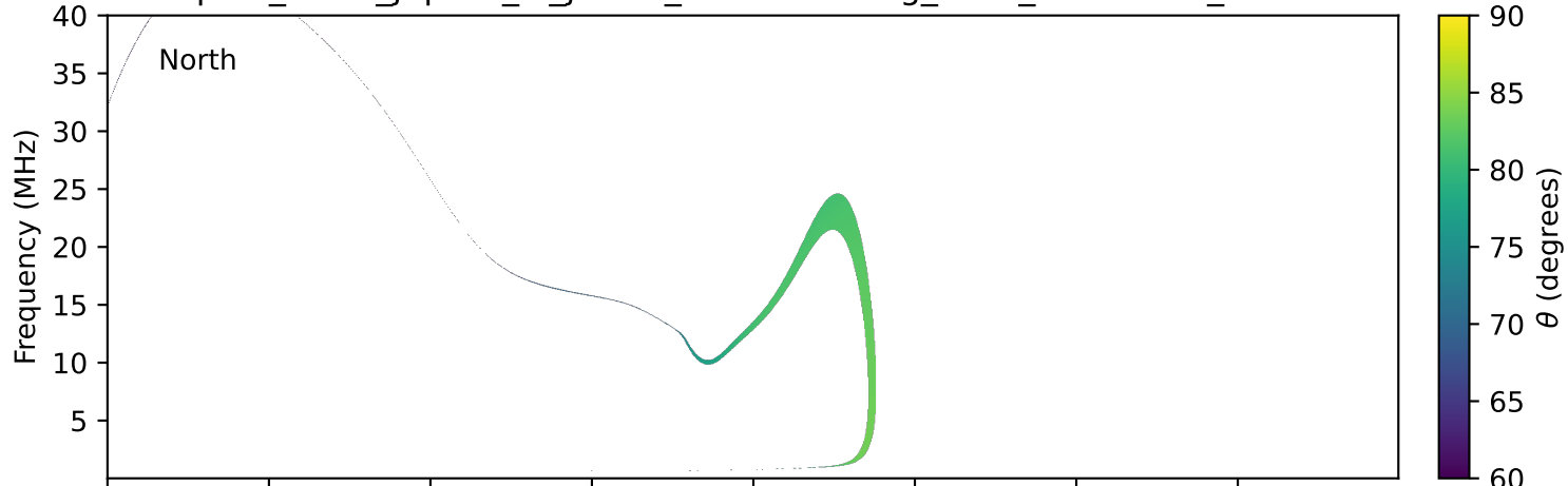
expres_earth_jupiter_io_jrm09_lossc-wid1deg_3kev_20230209_v11.cdf
