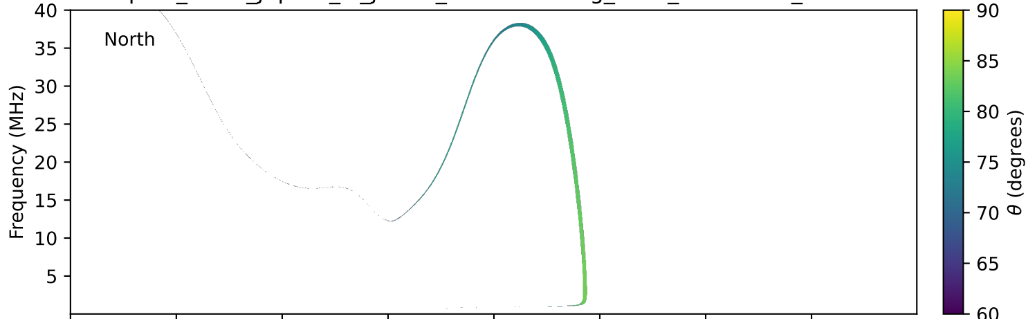
expres_earth_jupiter_io_jrm33_lossc-wid1deg_3kev_20221209_v11.cdf
