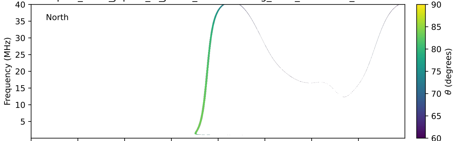
expres_earth_jupiter_io_jrm33_lossc-wid1deg_3kev_20210209_v11.cdf
