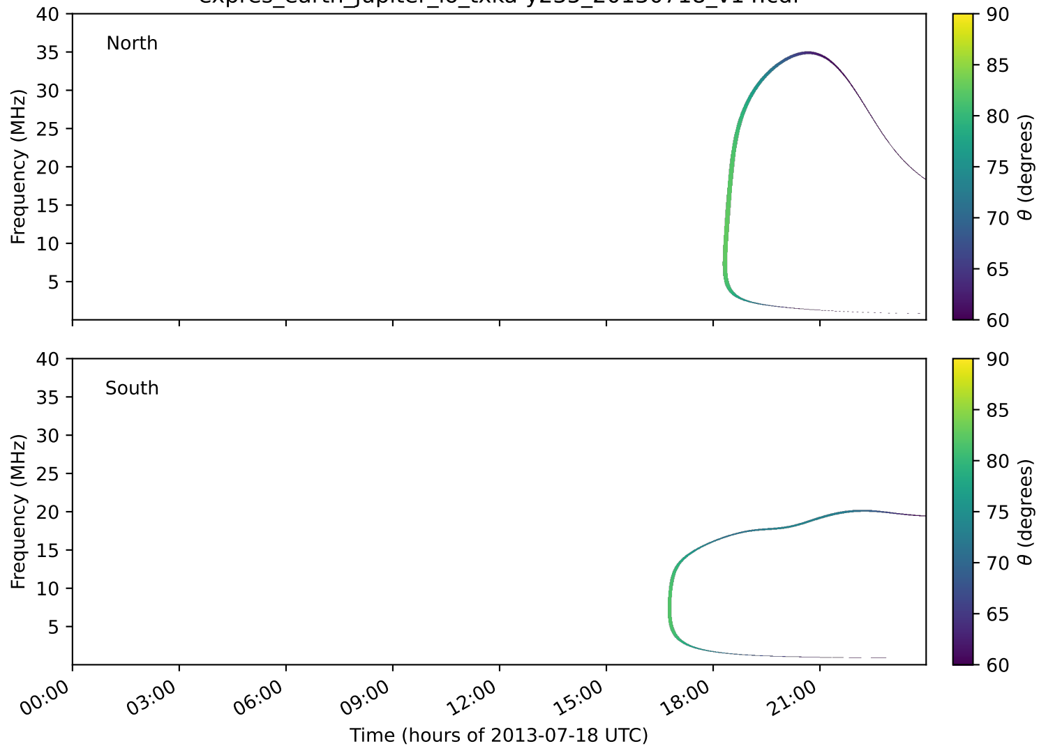
expres_earth_jupiter_io_txka-y235_20130718_v14.cdf
