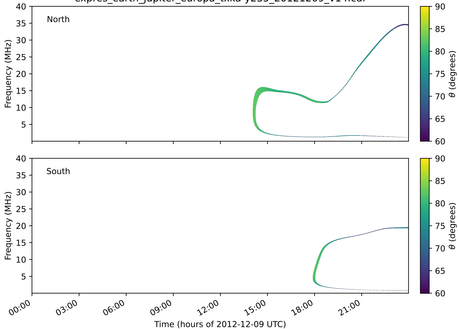
expres_earth_jupiter_europa_txka-y235_20121209_v14.cdf
