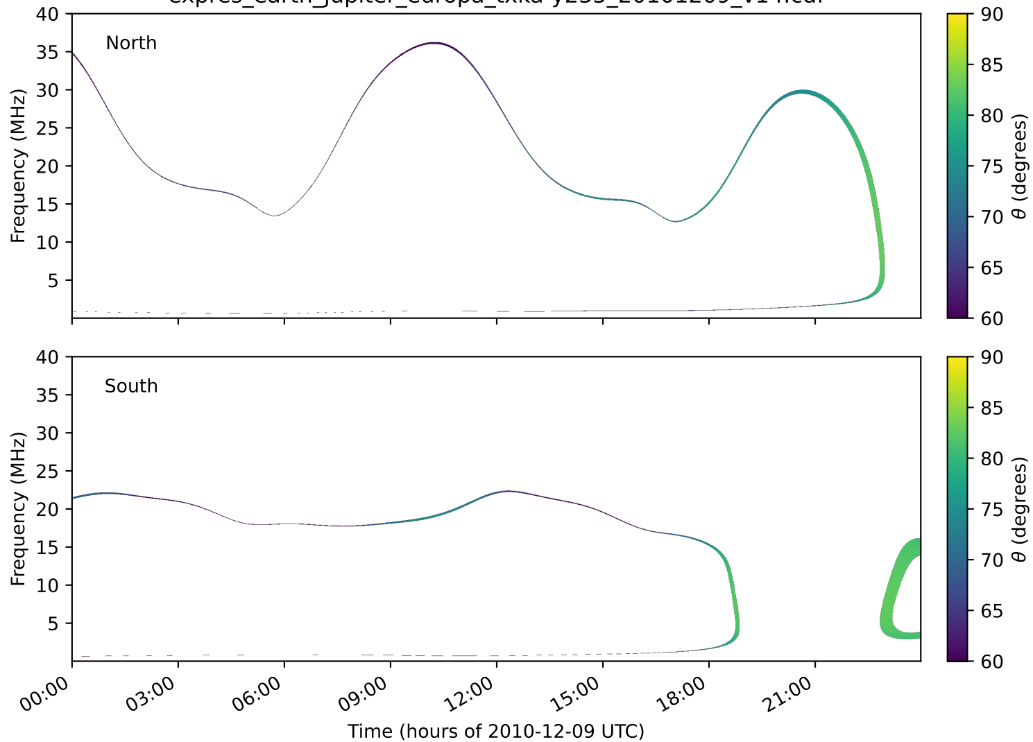
expres_earth_jupiter_europa_txka-y235_20101209_v14.cdf
